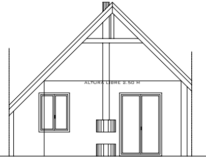
SECCIÓN AA'
