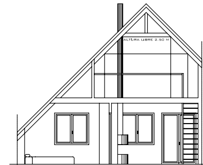
SECCIÓN CC'
