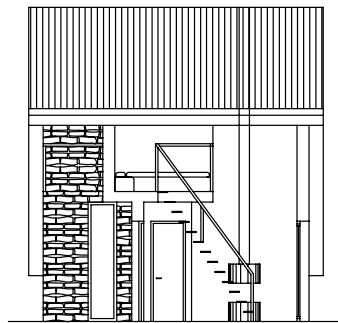
SECCIÓN BB'
