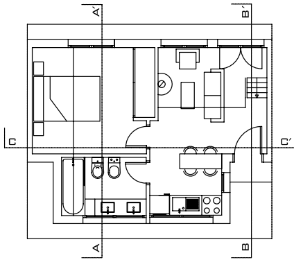
PLANTA BAJA
